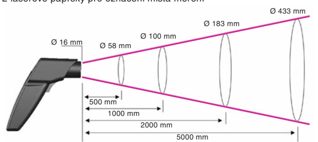
testo 830-T4
